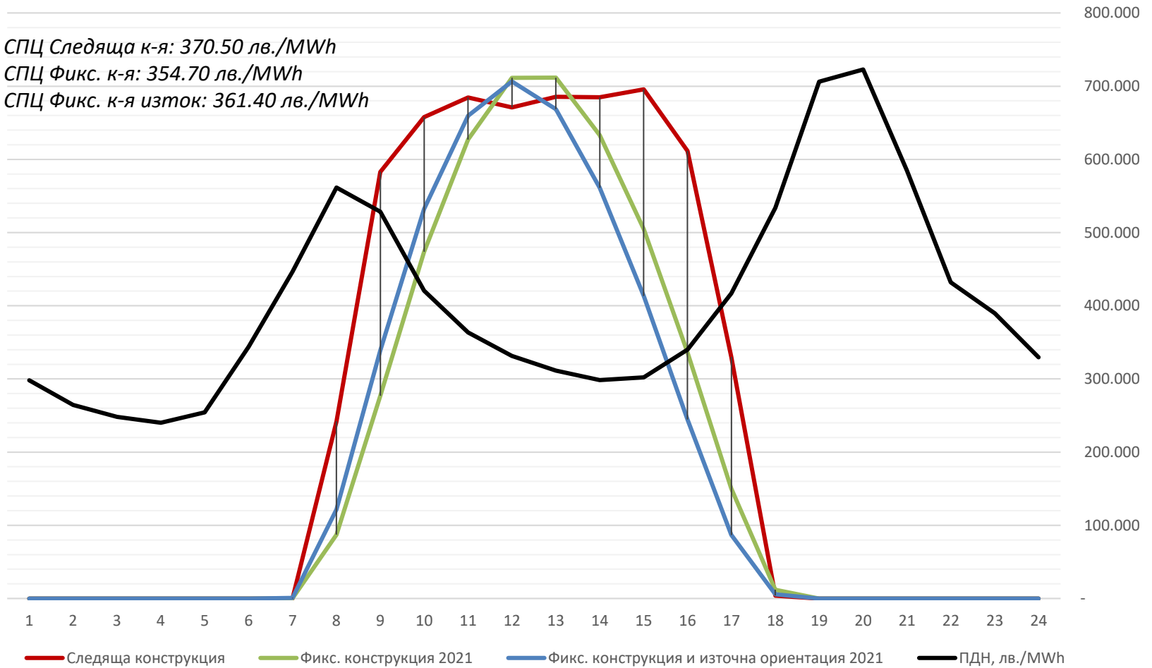
Сравнение между типове ФТЕЦ с БНЕБ, м. октомври 2022 г.
