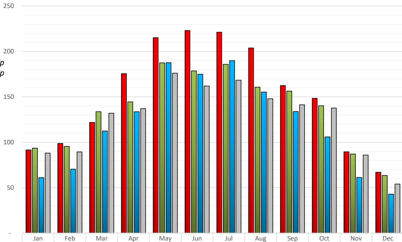
Добив на различните типове ФтЕЦ, kWh/kWp
